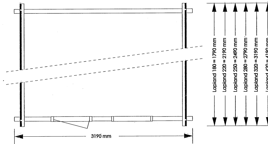
Plattegrond
