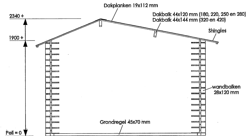
Doorsnede
