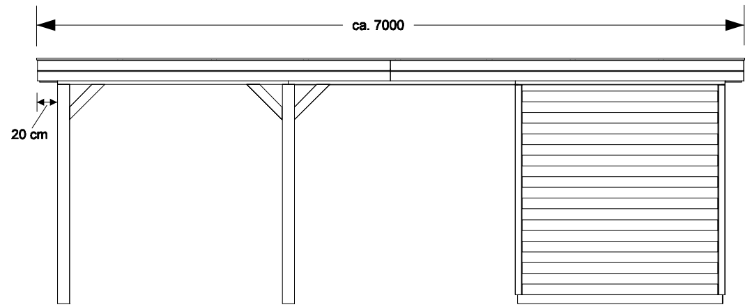
ACHTERAANZICHT
