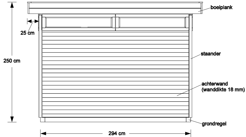
Achteraanzicht
