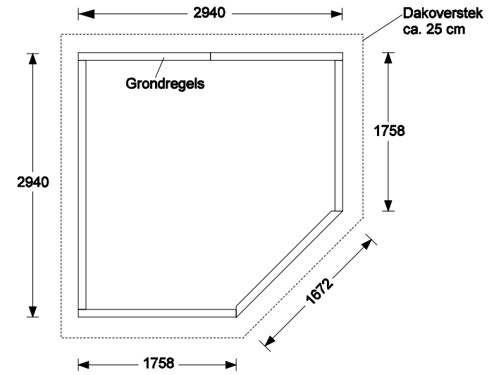
Plattegrond
